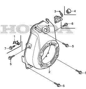
FAN COVER
