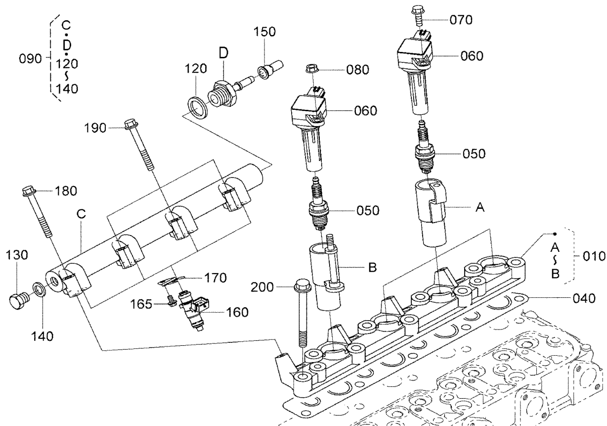
EG526-010-12
