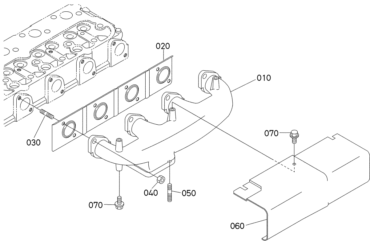
EG525-042-10
