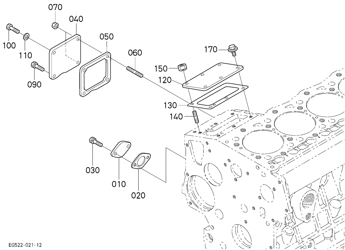
EG522-021-12
